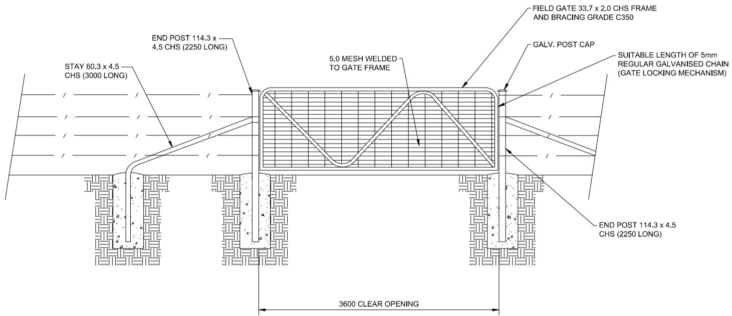
FIELD GATE DETAIL N.T.S
